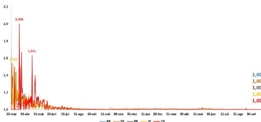
Figura 24 – Efeito da transmissibilidade
